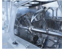
梨刀式
